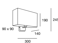
Ref 1703 1x 6w
