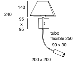
Ref 1700 1x 1,4w LED 1x 6w
