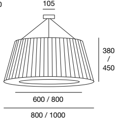
Ref 6937- 80 /100 5 x 9W
