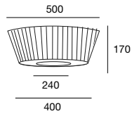
Ref 3400 2 x 9W
