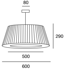
Ref 6937- 60 3 x 9W
