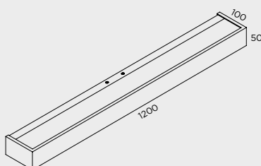
A-811/120 1 x T5 54W IP20
