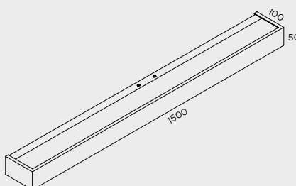
A-811/150 1 x T5 80W IP20
