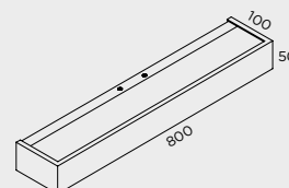
A-811/80 2 x T5 24W IP20
